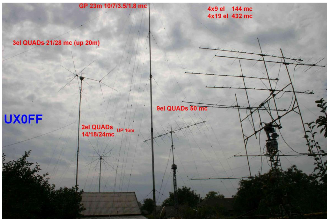
Общий вид антенн:
